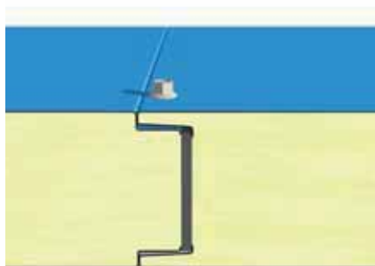
Modalità di fissaggio dei pannelli
